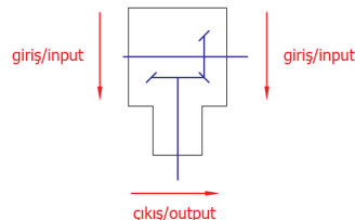
DIŞLI DÜZENİ / GEAR ARRANGEMENT
